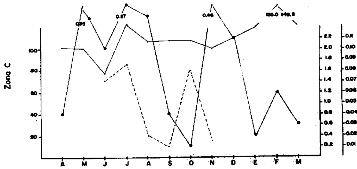
Fig. 5. Variación de los valores de conductividad, nitratos y fosfatos a lo largo de un año de estudio en las tres estaciones.
