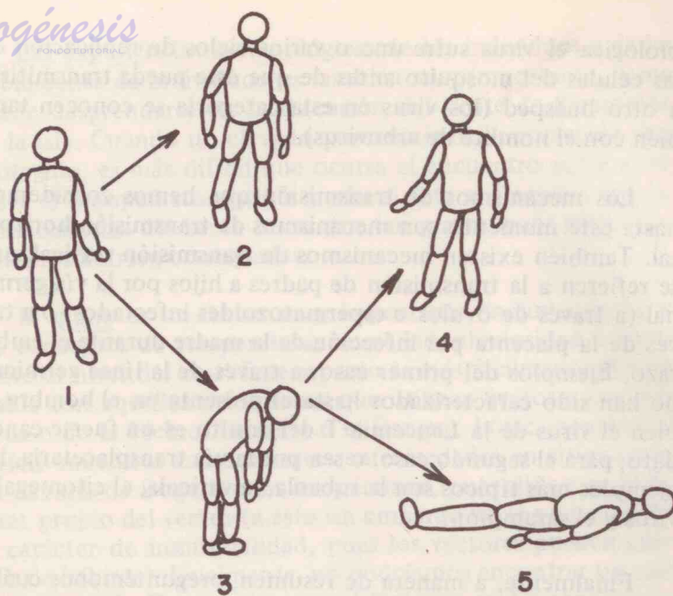
Fig.1 Posibles eventos en interacción de un virus con un huésped susceptible. Los individuos 2 y 3 son transmisores del virus a corto plazo, mientras sufren la infección subclínica y clínica respectivamente. A largo plazo, los individuos 2 y 4 pueden ser los reservorios del virus si se trata de infecciones crónicas (latentes o persistentes).
