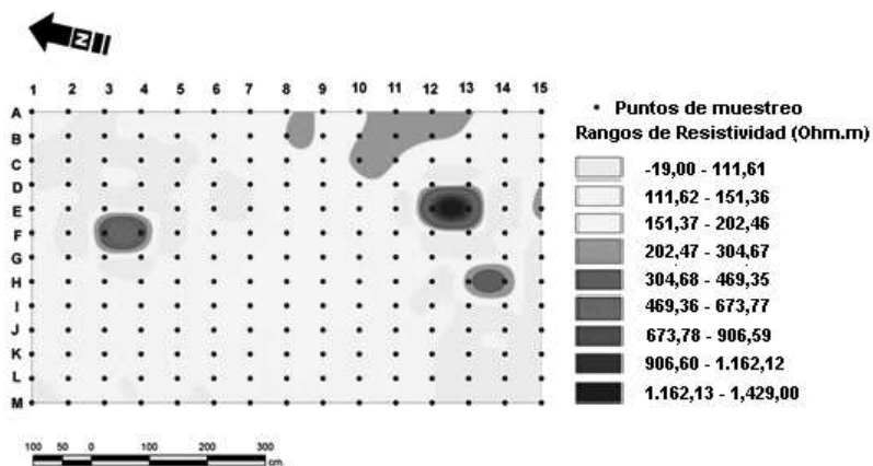
Figura 3. Mapa que muestra la distribución espacial de rangos de resistividad tomografía eléctrica en la Terraza 1
