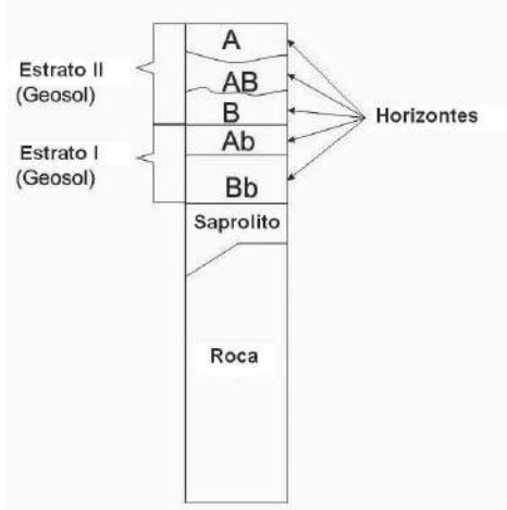
Figura 1. Columna pedoestratigráfica
