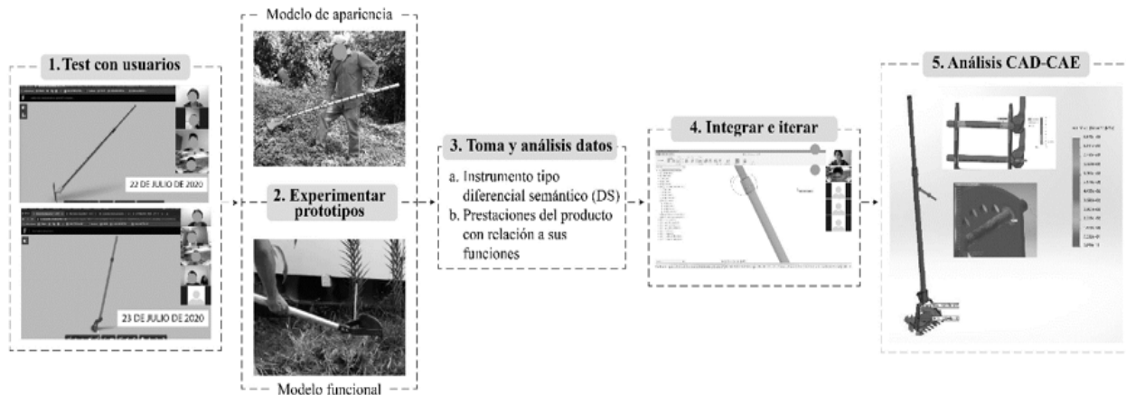
Figura 4. Proceso llevado a cabo para la verificación de una nueva propuesta de azadón. CAD-CAE: Computer Aided Design & Computer Aided Engineering.
