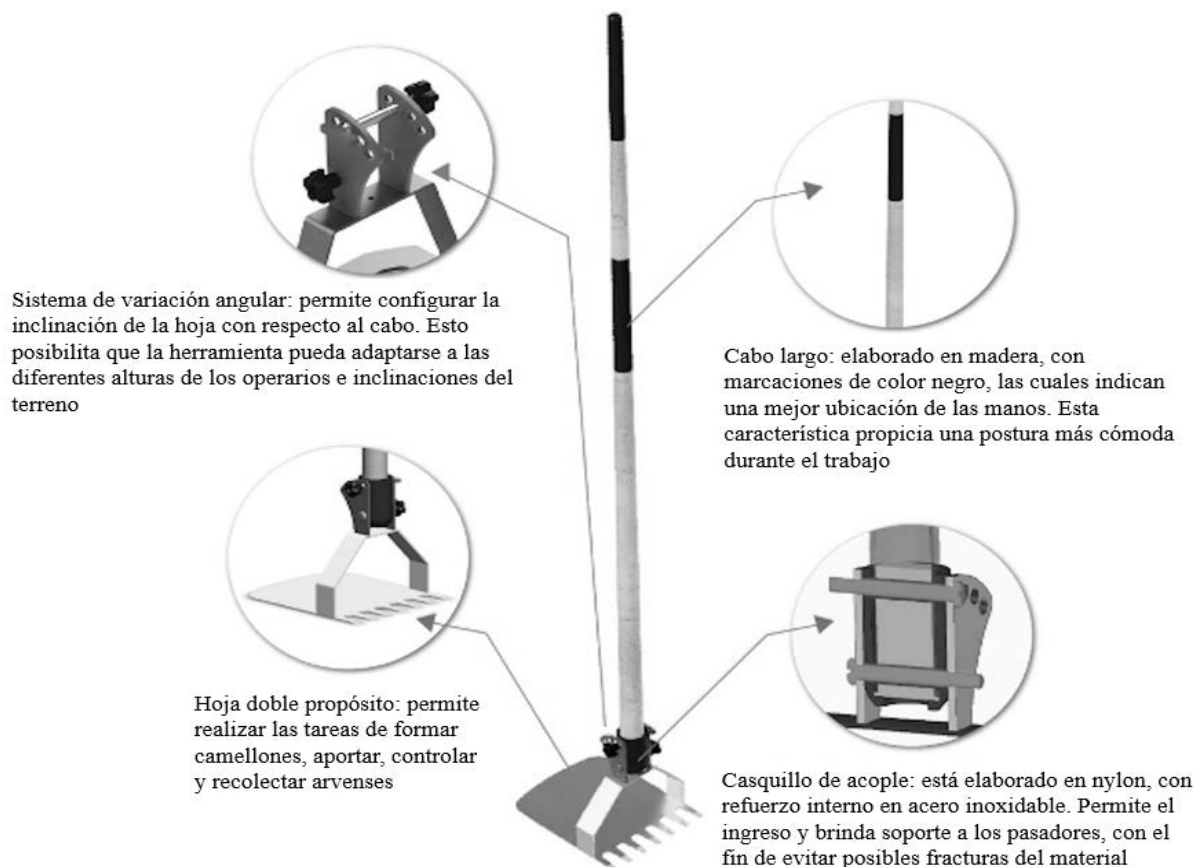
Figura 5. Nueva propuesta de herramienta manual de tipo azadón. En proceso de patentación.
