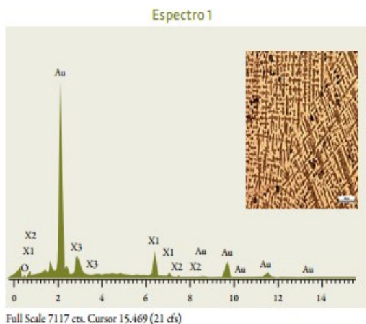
Figura 2. Ensayo SEM-EDS y micrografía que muestra estructura dendrítica en una de las gemas de oro de colores.
