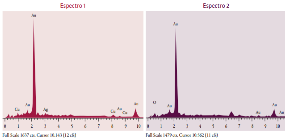
Figura 5. Ensayo SEM-EDS para el sistema cobre, plata, oro, cobre, obtenido por difusión
