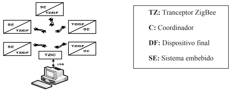
Figura 1 Diagrama de bloques del sistema
