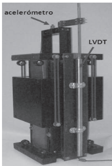
Figura 3 Actuador con LVDT y acelerómetro
