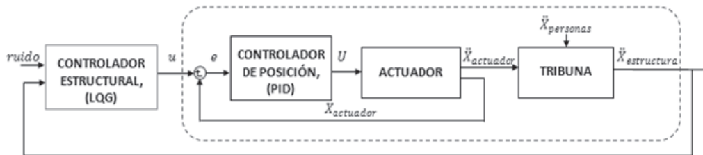
Figura 5 Diagrama de bloques detallado del sistema
