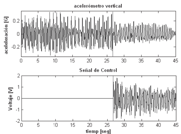
Figura 13 Respuesta de la estructura con y sin control durante el mismo ensayo
