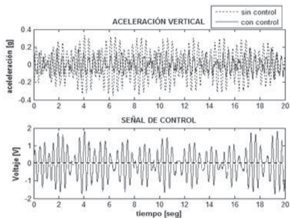
Figura 10 Respuesta de la estructura con y sin control ante una persona saltando
