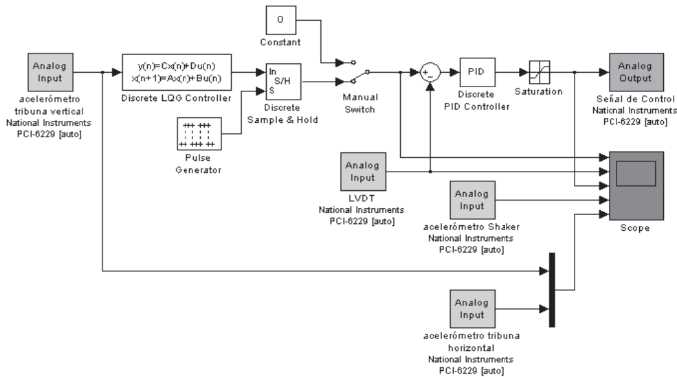
Figura 8 Implementación en SIMULINK del sistema de control activo
