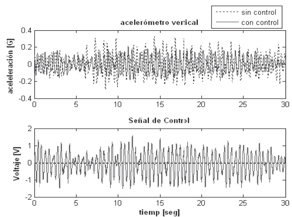
Figura 12 Respuesta de la estructura con y sin control ante tres personas saltando
