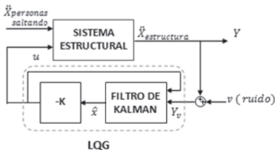
Figura 6 Diagrama de bloques del sistema estructural con el controlador
