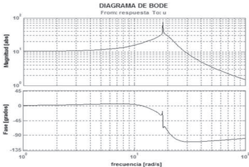
Figura 7 Respuesta en frecuencia del controlador LQG
