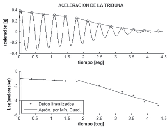
Figura 14 a.) Vibración libre con y sin control. b.) Linealización de los datos para determinar el amortiguamiento
