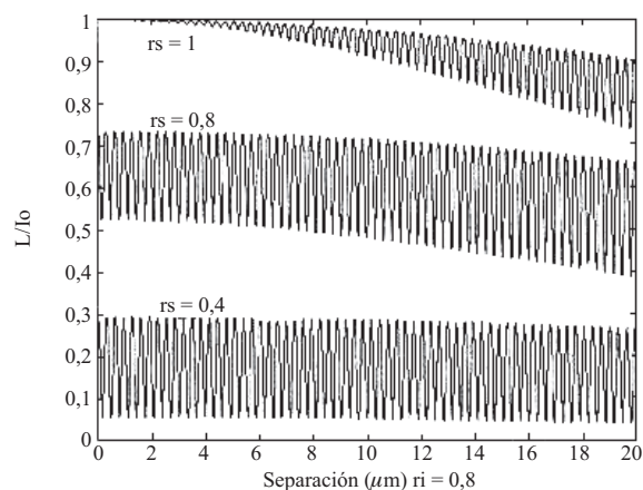
Figura 4 Intensidad reflejada en función del gap fibra-superficie reflectora. ( \lambda = 0,633 \mu\text{m} , r_{\text{int}} = 0,18 , w = 3\mu\text{m} )
