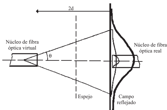
Figura 3 Efecto de la inserción de potencia en la fibra óptica al aumentar la distancia fibra-reflecto
