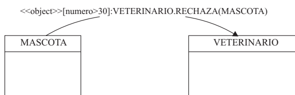
Figura 6 Diagrama de Interacción de objetos obtenido a partir del EP de la figura 5
