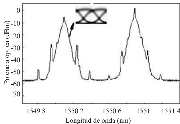
Figura 9 Espectros de los dos canales después de las etapas de conversión de longitud de onda
