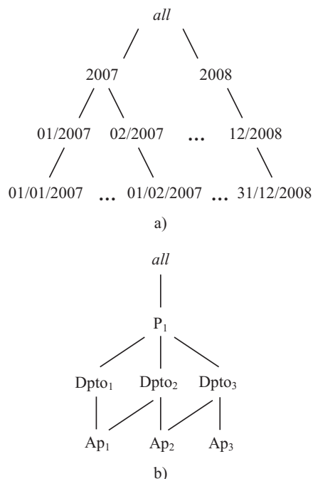
Figura 5 Instancias de dimensión: a) tiempo y b) ubicación
