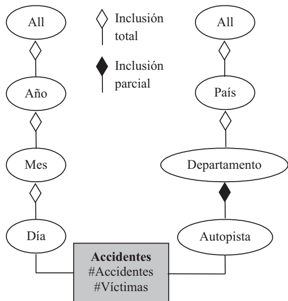
Figura 2 Modelo multidimensional para el análisis de accidentes
