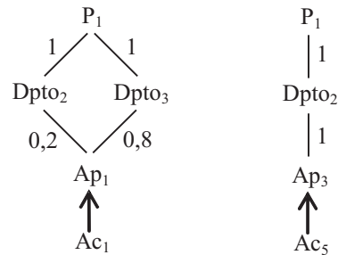
Figura 6 Hechos Ac_1 y Ac_5 asociados con valores dimensionales
