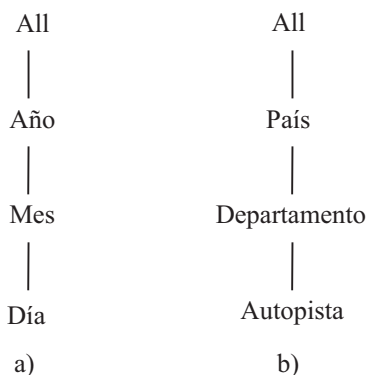
Figura 4 Orden parcial: a) dimensión Tiempo y b) dimensión Ubicación
