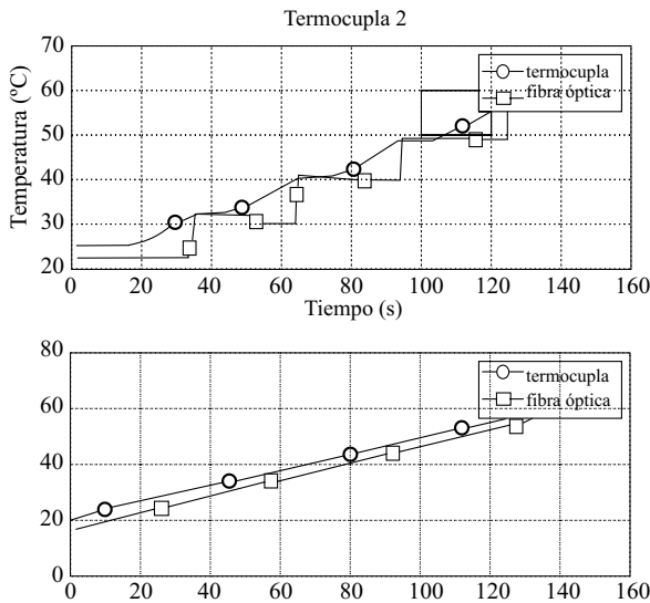
Figura 7 Ejemplo de curva de calibración de una termocupla
