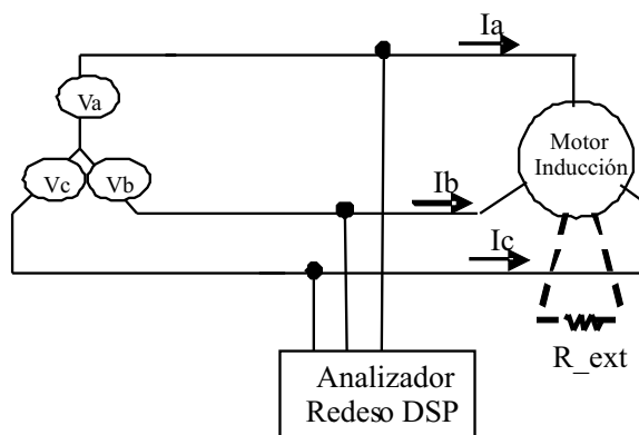
Figura 10 Montaje experimental
