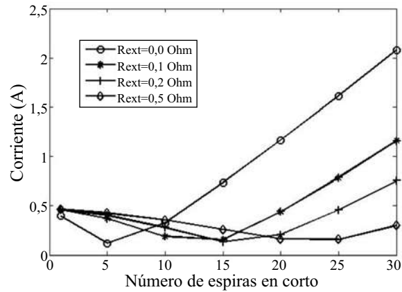
Figura 5 In versus el número de espiras en cortocircuito, plena carga y con desbalance de voltaje del 2,8%
