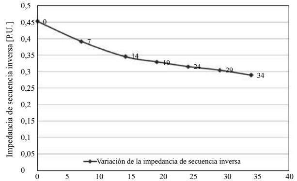
Figura 11 Impedancia de Secuencia Inversa para el motor con varias espiras en corto circuito (1740 rpm)
