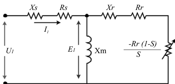
Figura 3 Circuito equivalente de secuencia inversa
