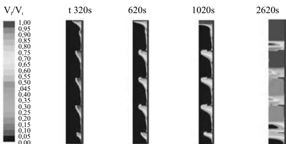
Figura 2a Fracción fundida para un intercambiador con aletas
