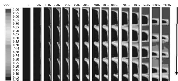
Figura 3a Fracción líquida T_{\text{aceite}} = 425\text{K} con g = 9,81\text{m/s}^2
