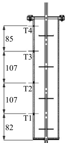
Figura 5 Puntos de medida de temperatura
