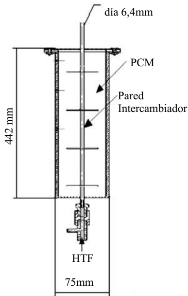
Figura 1. Esquema del sistema de almacenamiento de energía
