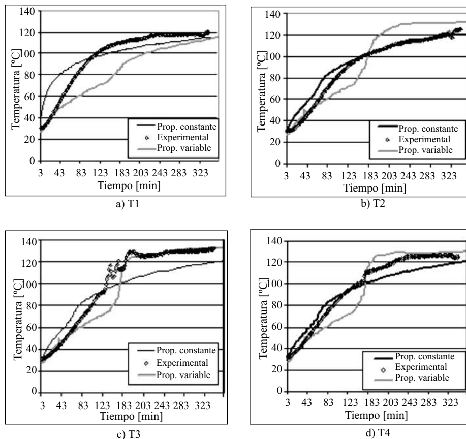
Figura 6 Validación del modelo teórico con resultados experimentales
