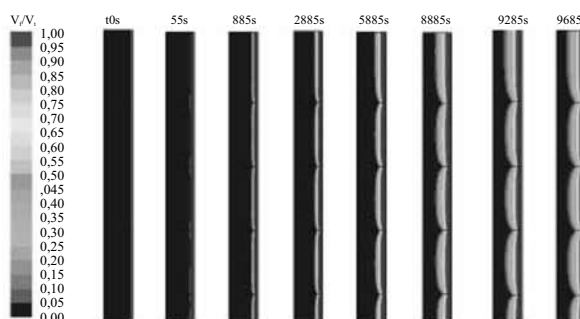
Figura 3b Fracción líquida T_{\text{aceite}} = 425\text{K} con g = 0 \text{ m/s}^2
