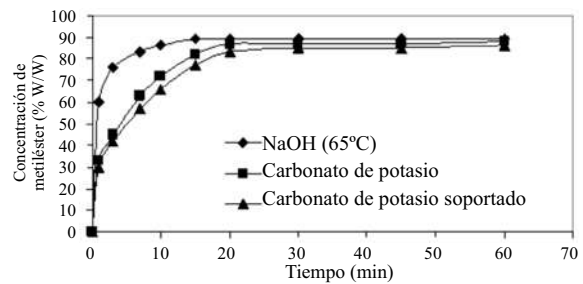
Figura 4 Transesterificación catalizadores homogéneos y heterogéneos a 65 °C
