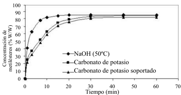
Figura 3 Transesterificación catalizadores homogéneos y heterogéneos a 50°C
