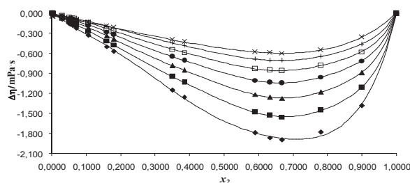
Figura 1 Desviaciones de viscosidad como función de la fracción molar de 1-pentanol para mezclas de 1-Pentanol en DMF a las temperaturas de ◆283,15; ■288,15; ▲ 293,15; ●298,15; □303,15, +308,15, x313,15 K.
