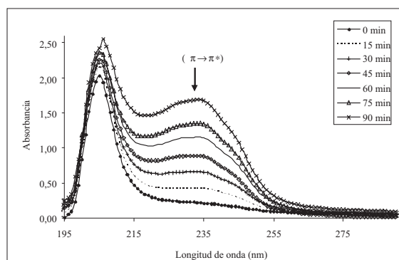
Figura 5 Espectros de absorción del linoletato de metilo y de los hidroperóxidos formados en la reacción con oxígeno singlete generado por el sistema Na_2MoO_4/H_2O_2
