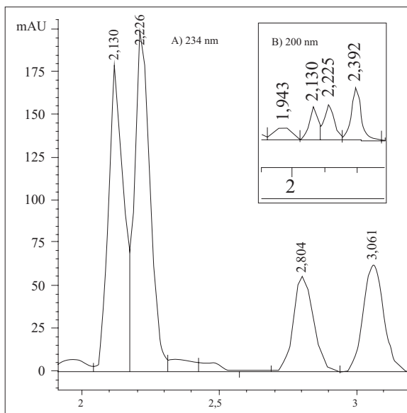
Figura 6 Cromatograma HPLC de los productos de oxidación del linoleato de metilo. A) 234 nm, B) 200 nm
