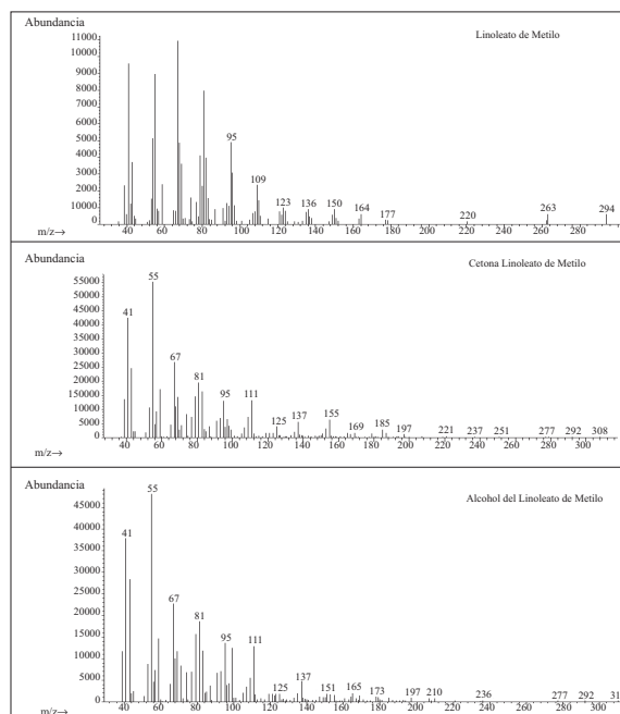
Figura 7 Espectro de masas del linoleato de metilo, del alcohol y su cetona
