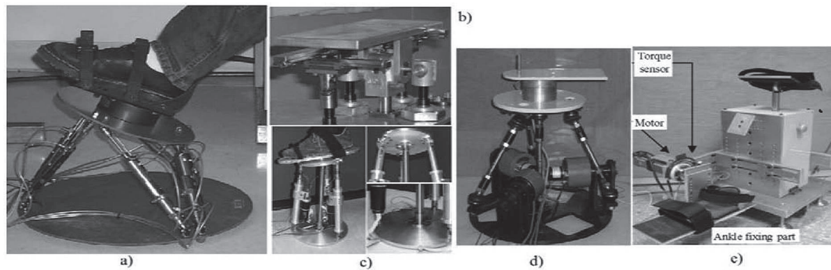
Figura 3 Rehabilitadores para tobillo a) - d) basados en mecanismos paralelos y e) de 1 gdl
