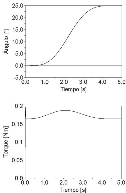
Figura 10 Ángulo de dorsiflexión y torque requerido implementando un control PID - prototipo virtual
