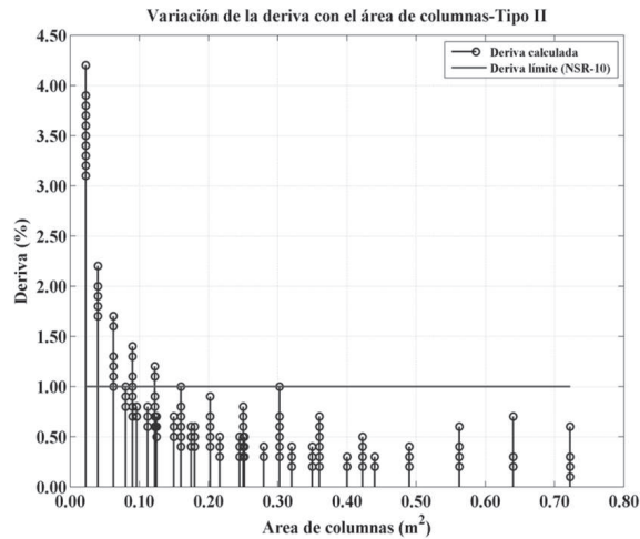
Figura 7 Variación de deriva para un mismo valor de sección de columna (modelos de 3 pisos)
