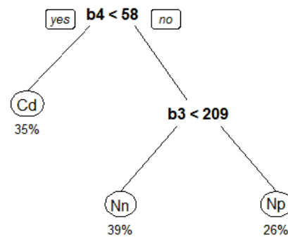
Figura 4 Reglas del árbol de decisión
