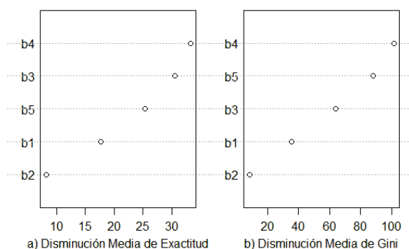
Figura 5 Medidas de importancia de las bandas
