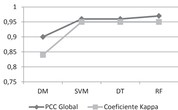
Figura 8 Medidas de exactitud por método
