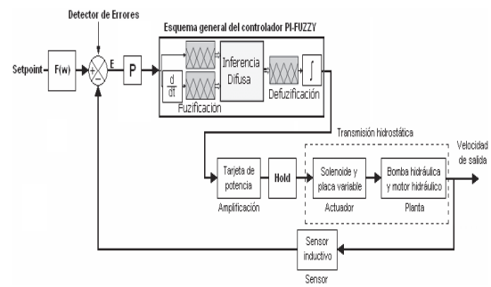
Figura 7 Diagrama de bloques del sistema
