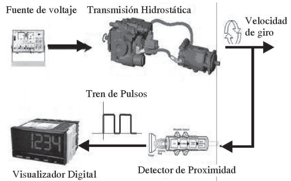
Figura 3 Montaje para obtención de datos de las pruebas de lazo abierto
