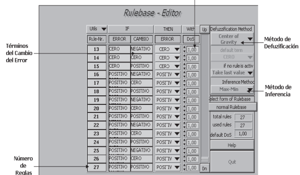
Figura 11 Reglas del controlador
