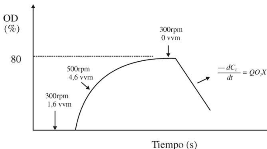
Figura 3 Variación de la concentración de OD en un cultivo de Ganoderma lucidum durante la determinación del QO_2
