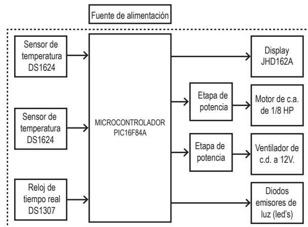
Figura 4 Diagrama de bloques del sistema de control
