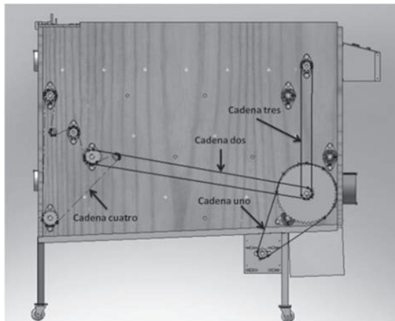
Figura 3 Vista frontal del prototipo
