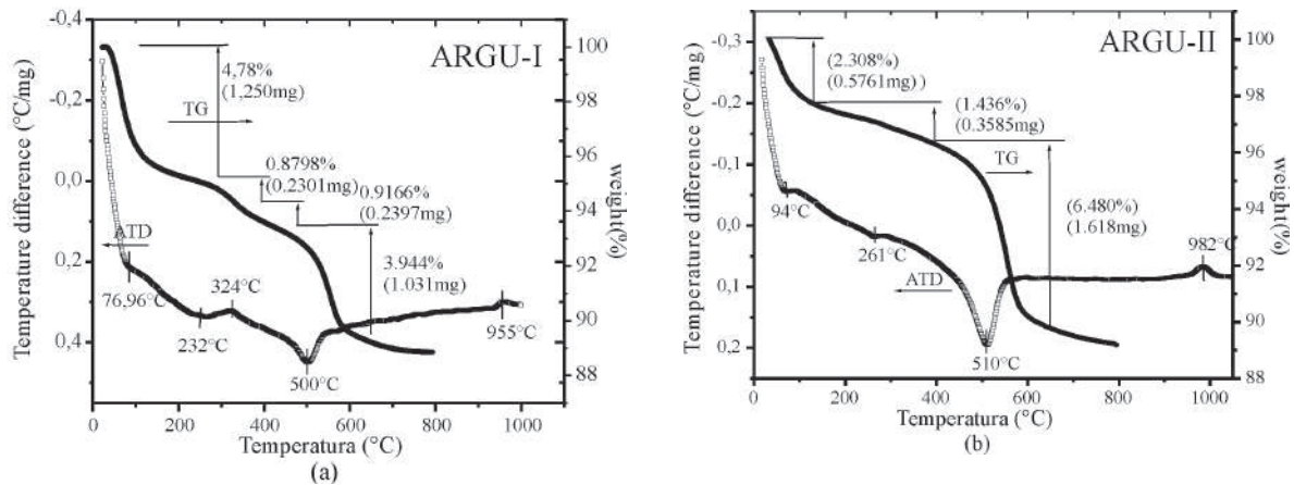
Figura 3 Curvas de ATD/TG correspondientes a: a) ARGU-I y b) ARGU-II
