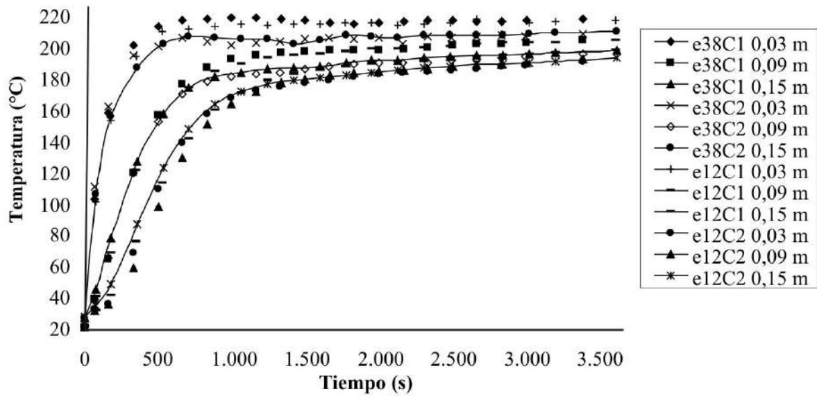
Figura 3 Curvas experimentales de calentamiento para esferas
