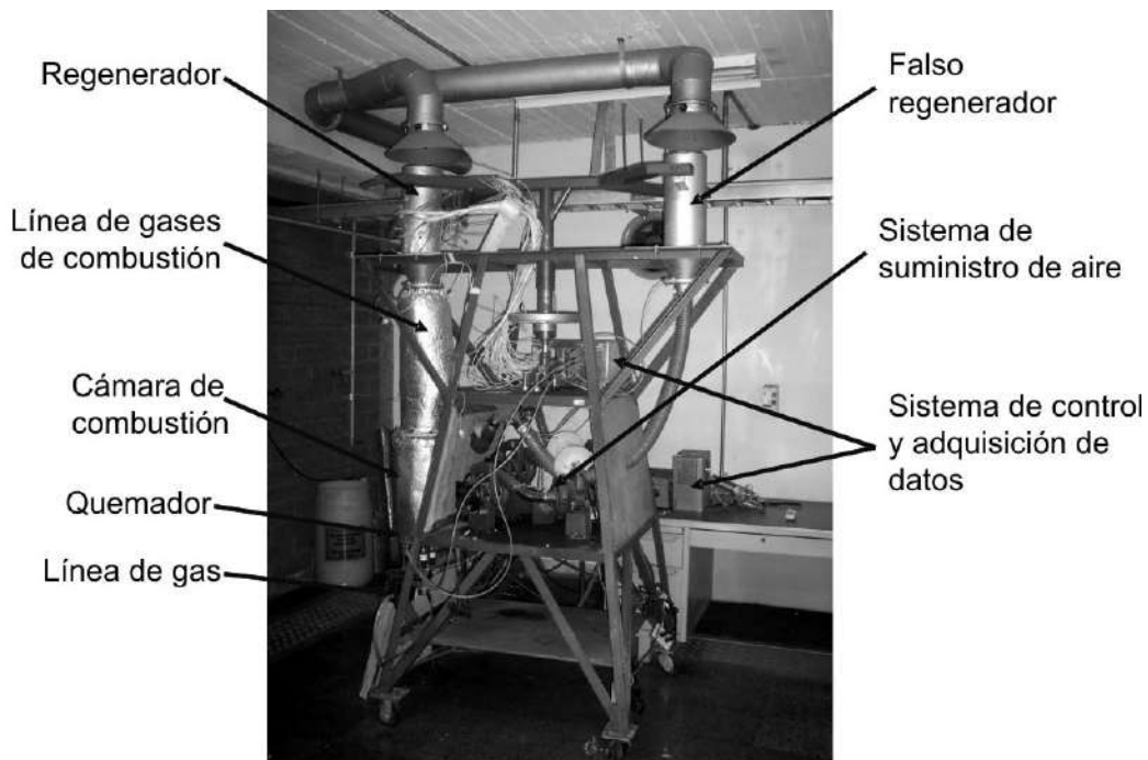
Figura 1 Banco de pruebas para regeneradores térmicos de lecho poroso empacado [4]
