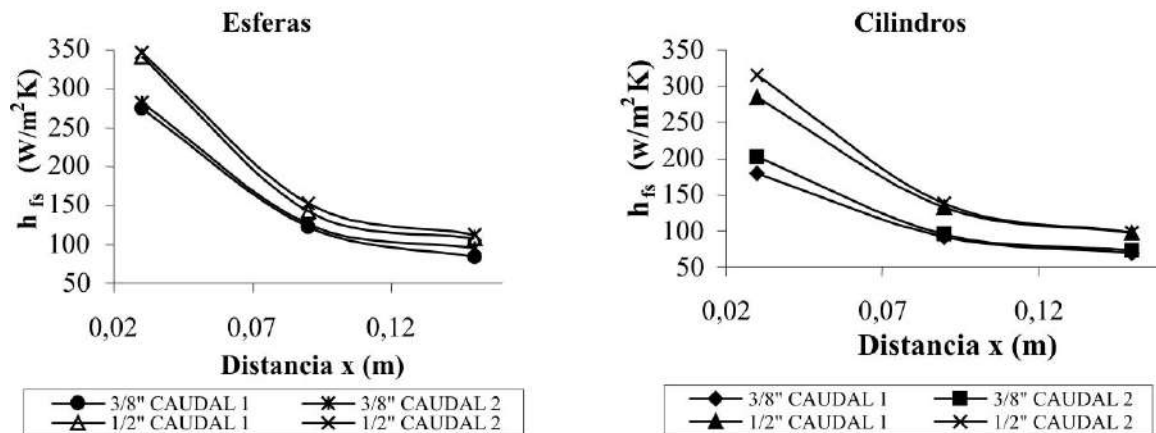
Figura 5 Coeficientes de convección fluido-sólido en función de la distancia x para esferas y cilindros
