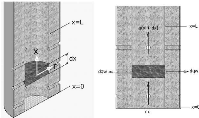
Figura 8 Representación esquemática del lecho poroso empaçado
