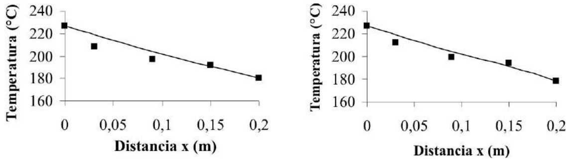
Figura 9 Comparación de las temperaturas de estado estable calculadas con las experimentales para esferas de 3/8" a caudal C2 (izquierda) y esferas de 1/2" a caudal C2 (derecha)
