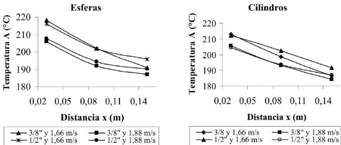
Figura 7 Distribución de temperatura axial en estado estable para esferas y cilindros
