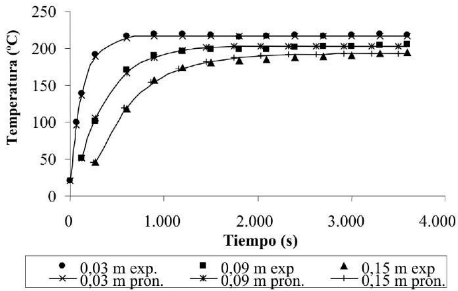
Figura 11 Comparación entre los valores obtenidos mediante la función de distribución de temperatura propuesta y los datos experimentales para esferas de 3/8" y caudal C1; exp: mediciones experimentales, pron: predicciones del modelo
