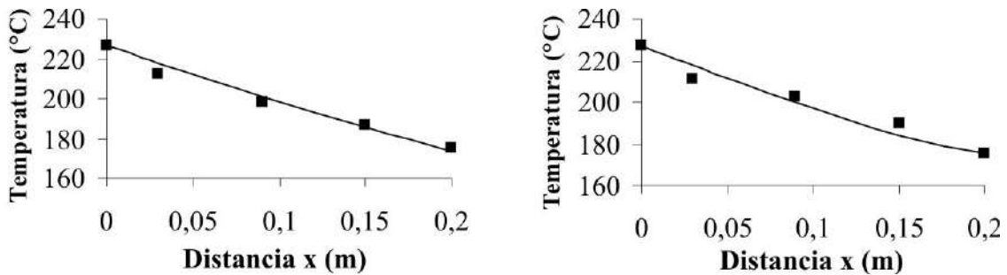
Figura 10 Comparación de las temperaturas de estado estable calculadas con las experimentales para cilindros de 3/8" a caudal C1 (izquierda) y cilindros de 3/8" a caudal C2 (derecha)
