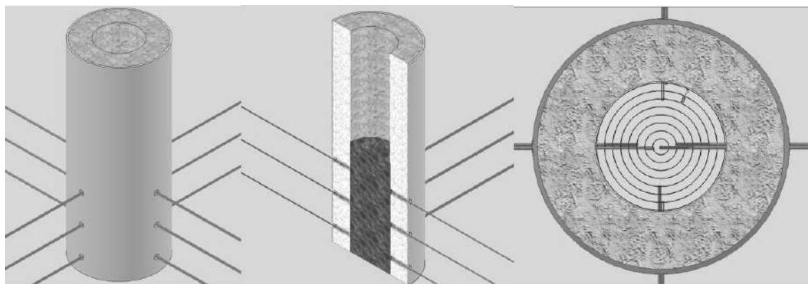
Figura 2 Distribución de termopares en el lecho poroso empacado
