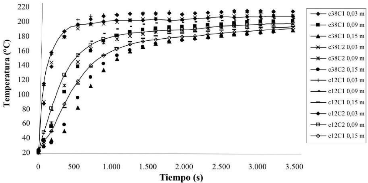
Figura 4 Curvas experimentales de calentamiento para cilindros
