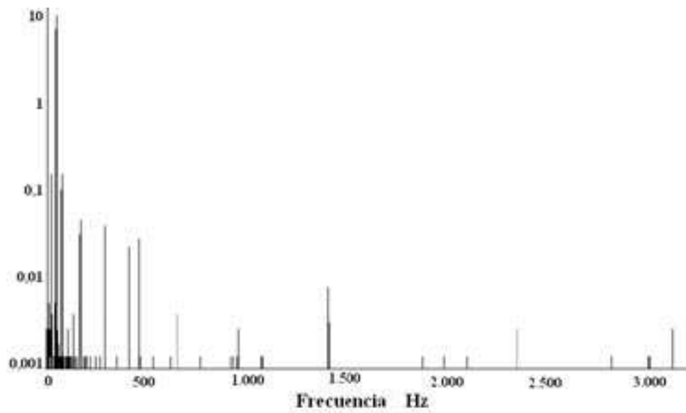
Figura 3 Espectro de corriente para 10 espiras del estator en cortocircuito
