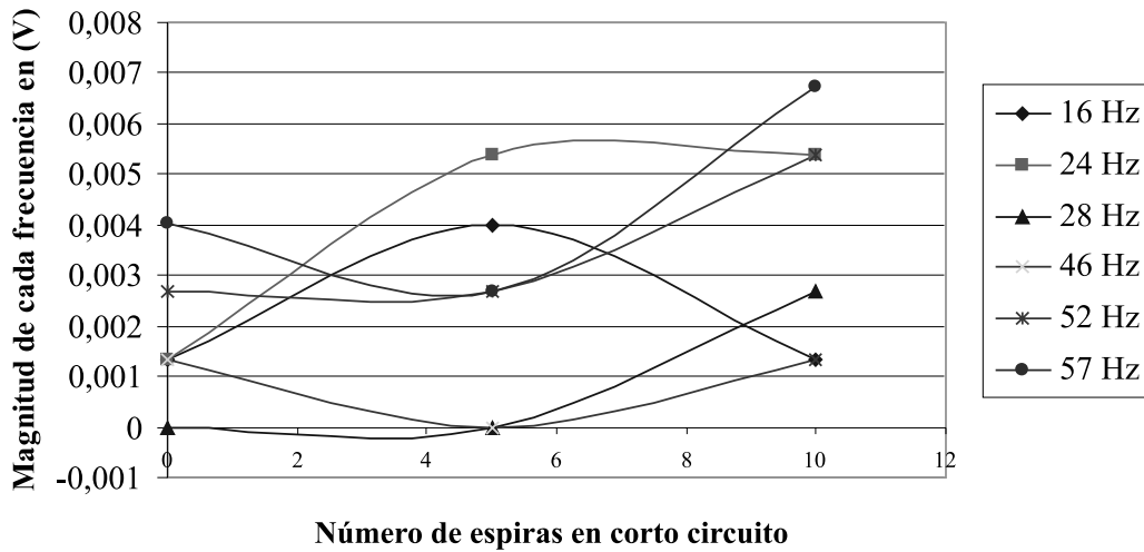
Figura 6 Variaciones en la amplitud de algunas frecuencias versus 5 y 10 espiras en cortocircuito
