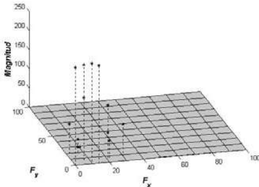
Figura 7 Coeficientes de Fourier en trozo defectuoso de urdimbre rota
