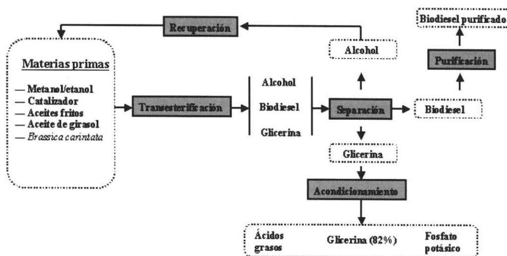
Figura 2 Esquema de producción de biodiesel. Método de la Universidad Complutense de Madrid y el Instituto para la Diversificación y Ahorro de la Energía —IDAE— [1]
