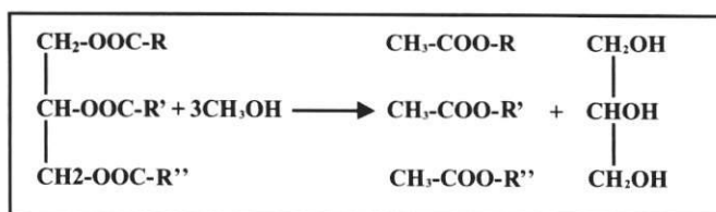
Figura 1 Vista esquemática de la reacción de transesterificación: el triglicérido reacciona con el alcohol (metanol) para producir ésteres y glicerina
