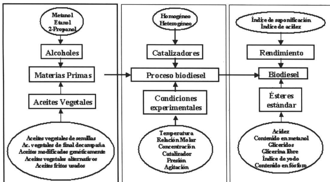
Figura 3 Diagrama de bloques de la producción de biodiesel [1]
