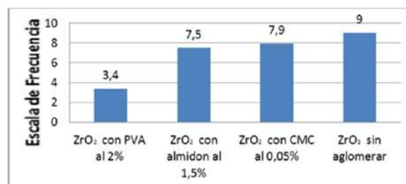
Figura 5. Evaluación de la fluidez de los aglomerados, a partir de la frecuencia de vibración en el alimentador de polvos de la antorcha de proyección térmica
