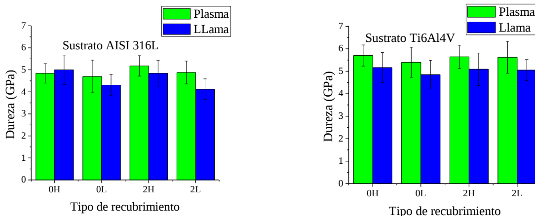
Figura 2. Dureza de los recubrimientos de vidrio bioactivo Vs técnica de proyección
