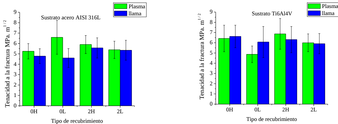
Figura 3. Tenacidad a la fractura de los recubrimientos de vidrio bioactivo vs técnica de proyección
