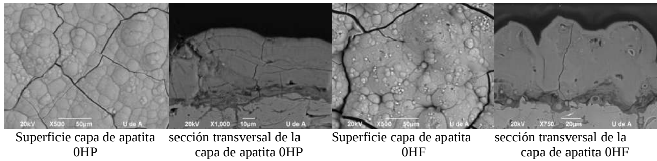
Figura 4. Micrografías SEM de la capa de apatita formada en los recubrimientos de vidrio bioactivo 0HP y 0HF después de 15 días de inmersión en SBF.
