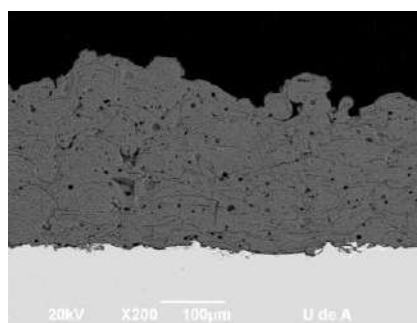
Figura 1. Micrografía SEM del recubrimiento 0HF elaborado por proyección térmica por llama
