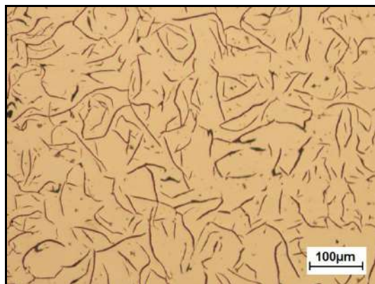
Figura 2. Microestructura del hierro gris inoculado con SiC. Tamaño de lámina de grafito libre N° 3. Probeta sin ataque metalográfico.
