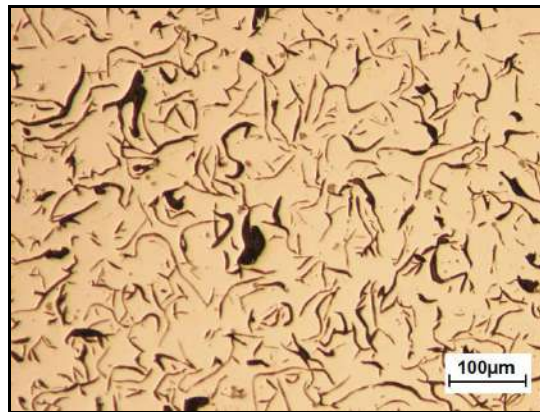
Figura 5. Microestructura del hierro gris sin inocular. Tamaño de lámina de grafito libre N° 6. Probeta sin ataque metalográfico.
