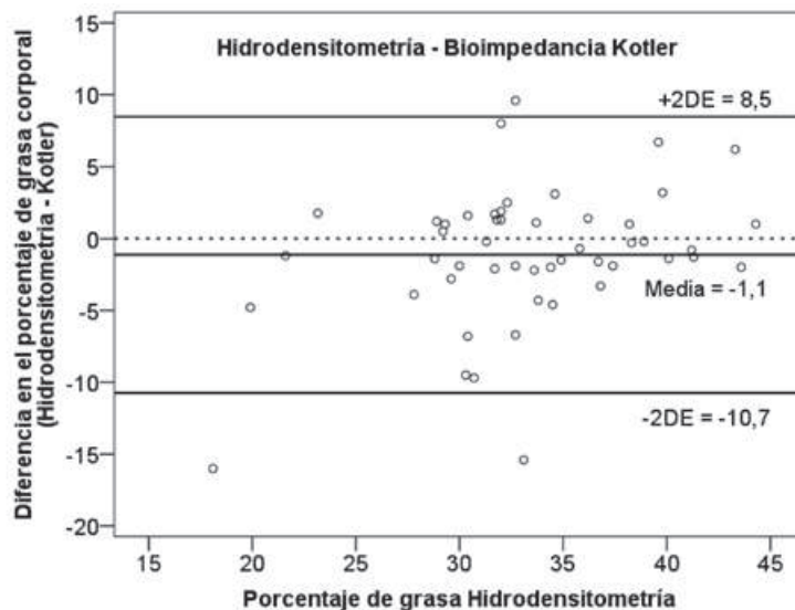
Figura 2. Concordancia del porcentaje de grasa corporal obtenido por hidrodensitometría y bioimpedancia mano-pie con la ecuación de Kotler.
