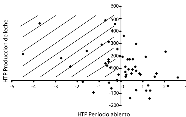
Figura 2. Ejemplo de NID con una fracción descartada del 72%, correspondientes a progresos genéticos de mínimo 0 Kg para producción de leche por lactancia y de máximo 0 días para los PA. Las líneas de los ejes X y Y en la figura representan la ubicación de los límites o NID para cada característica, de manera que los animales que se encuentran dentro del área con líneas transversales corresponden a los animales seleccionados.
