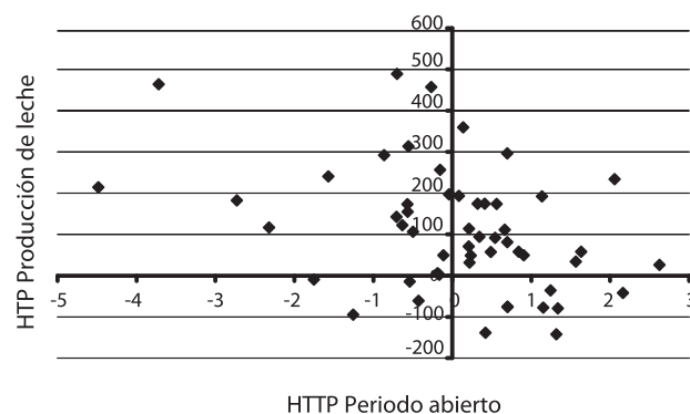
Figura 1. Distribución de la población en estudio según sus habilidades predichas de transmisión para producción de leche y periodo abierto.
