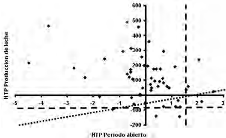
Figura 3. Representación de los animales seleccionados y descartados según cada uno de los métodos (NID, Índice), para una tasa de reemplazo del 25%.
