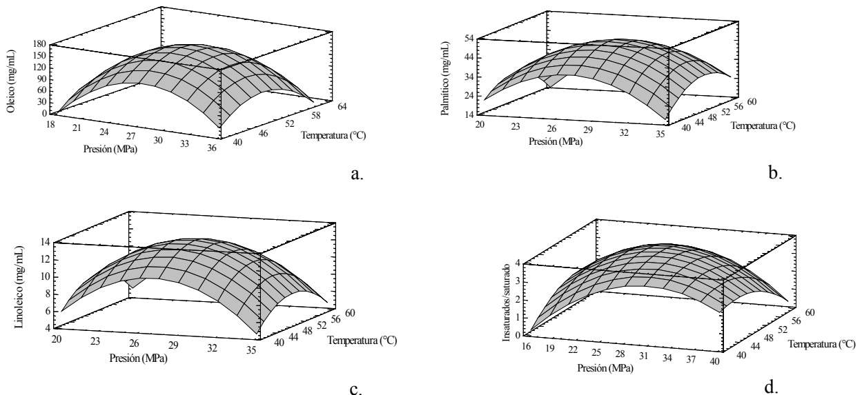
Figura 3. Superficie de respuesta para el efecto de la temperatura y presión sobre el contenido de: (a) ácido oleico, (b) ácido palmítico, (c) ácido linoleico y (d) relación de ácidos grasos insaturados/saturados.
