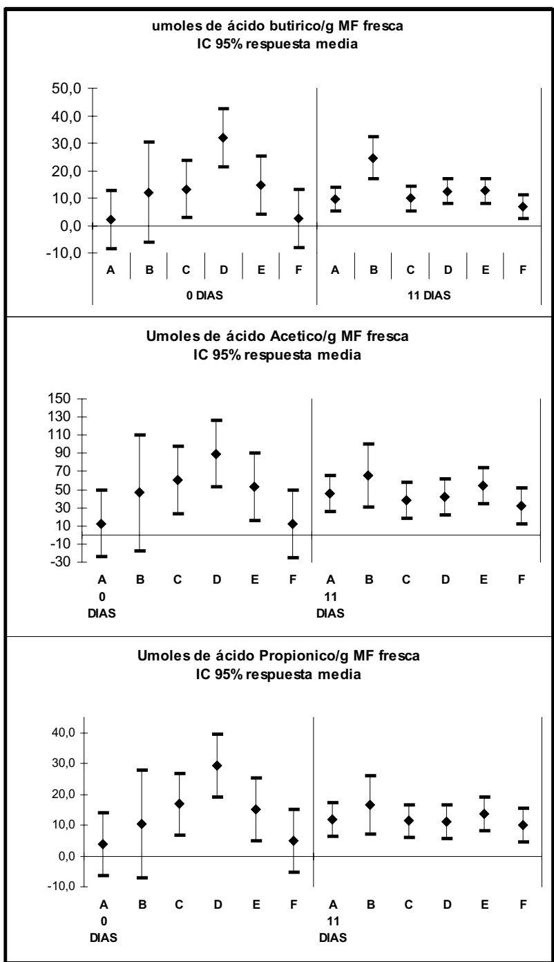
Figura 5. Respuesta media de ácido butírico, ácido acético y ácido propiónico ( \mu\text{moles/g} ).
