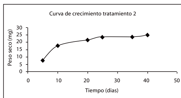
Figura 4. Curva de crecimiento en el medio seleccionado (Tratamiento 2)
